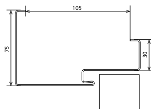
sarokrész - NAGY fém saroktok
