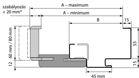
PROJEKT BIS tok metszet
