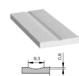
marás
