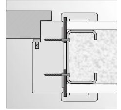
Beépítés csavarokkal gipszkarton falba
