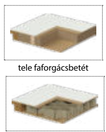
papírrácsbetét
