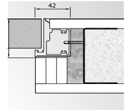
PORTA HIDE falc nélküli (kifelé nyíló)
