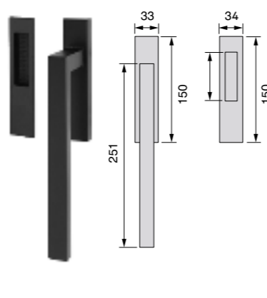
GL-1402PI/80KG, üveghez GL-1401I/80KG, fához központi toldóelem rúd, inox, 2x1db
