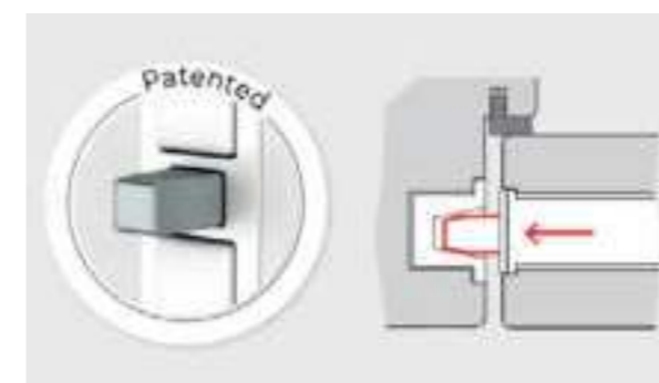
A toalett gomb vagy a kulcs elfordításakor előugró retesz rögzíti a tokhoz az ajtószárnyat.
