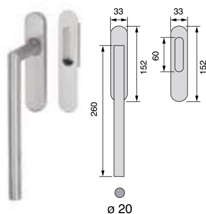
GL-1402PI/80KG, üveghez GL-1401I/80KG, fához központi toldóelem rúd, inox, 2x1db
