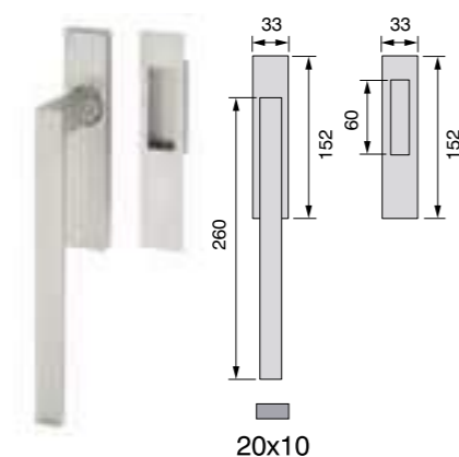
GL-1402PI/80KG, üveghez GL-1401I/80KG, fához központi toldóelem rúd, inox, 2x1db
