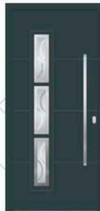
Modell/ Model MILANO Farbe RAL/ Ral colour 7026 Verglasung/ Glass DPM Applikation/ Application GEBÜSTET/ BRUSHED Griff/ Handle ACR 115h Rostzeit RRP 30
