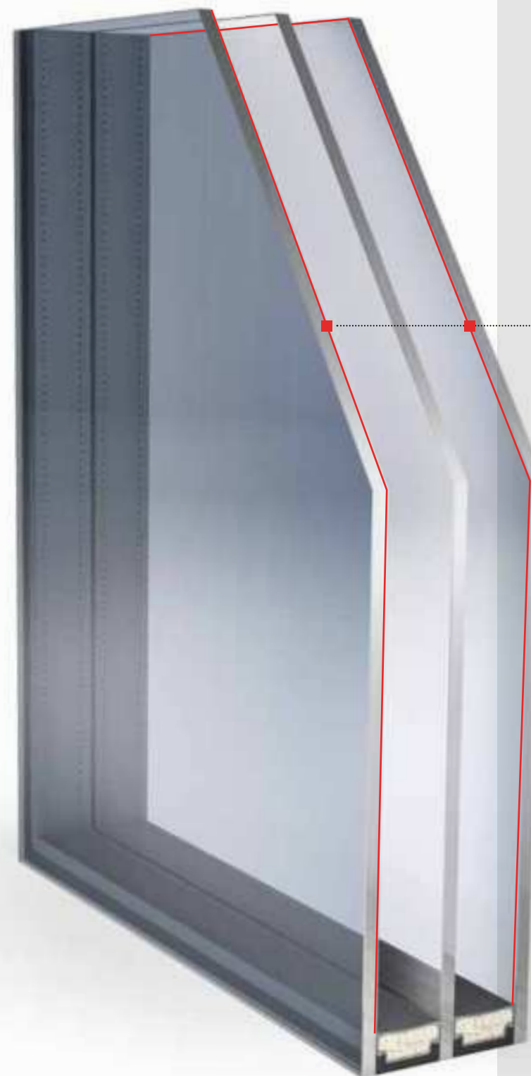
Példa: Szabványos háromtáblás hőszigetelő üveg két bevonattal
